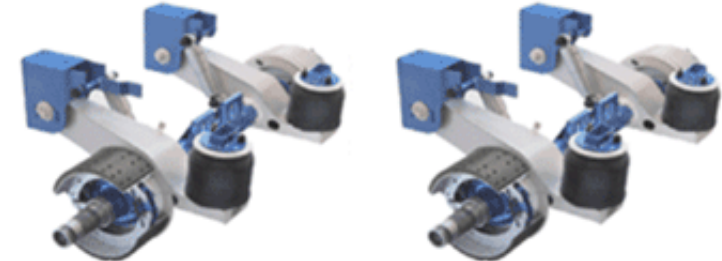
"Boggie" (normalmente em caminhões 6x4)
